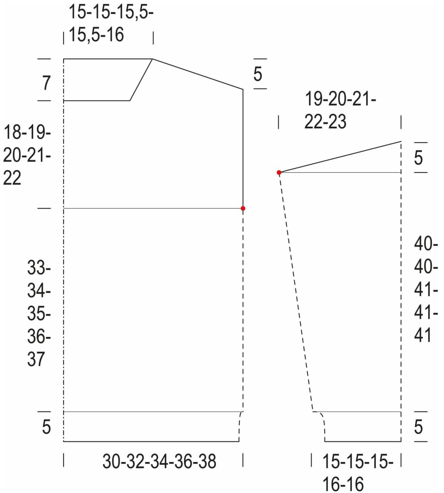
Выкройка свитера, см
